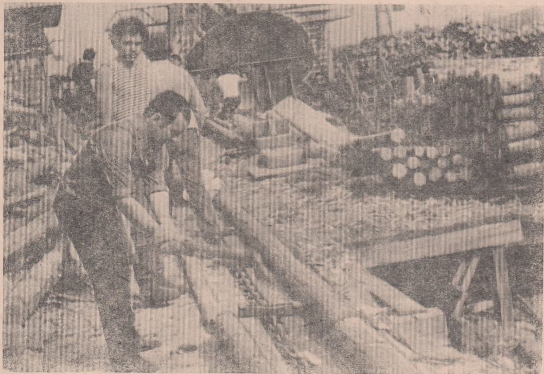
Нижний склад Дзержинского леспромхоза. Разделка леса ведется на полуавтоматической линии.
